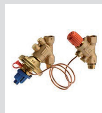
Automatischer Differenzdruckregler Kombi-Auto Kombi-SY
